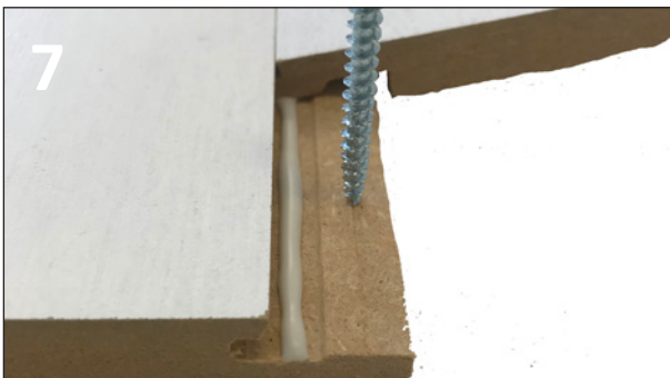
7 CA. 1 MM TYKK LIMSTRENG VINTERLIM NEDE I PROFILEN. BENYTT SPOR FOR SKRUE/KRAMPER.
