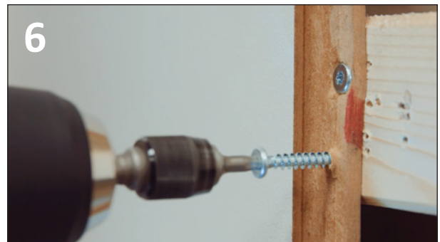
6 DOBBEL INNFESTING PÅ HORIZONTAL UTLEKTING.
