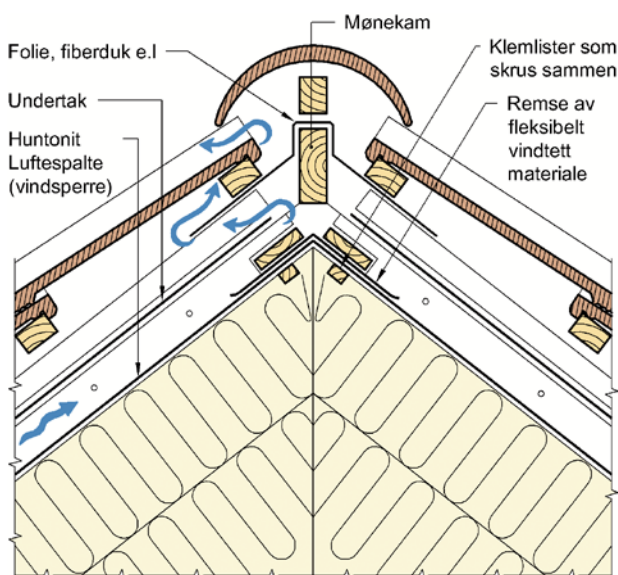
Fig. 4 Eksempel på mønedetalj. Overgangen mellom platene i de to takflatene skal gjøres lufttett ved å legge et rullbasert vindsperreprodukt som er klemt fast med klemlekt.
