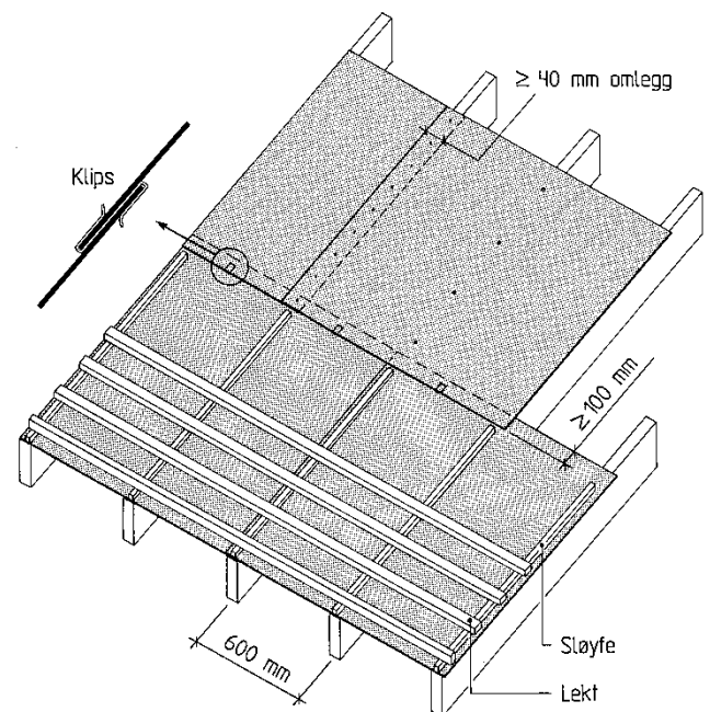
Fig. 1 Huntonit Sutak undertakplater legges i forband. Bruk av klips i plateskjøtene forenkler monteringen og reduserer faren for inndrev av regn- og snø.
