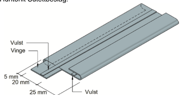
Fig. 2 Huntonit Sutettbeslag
