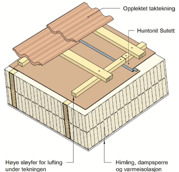
Fig. 1 Prinsipiell oppbygning av skrå tretak med Huntonit Sutett kombinert undertak og vindspærre alltid i forbindelse med Huntonit Sutettbeslag.
