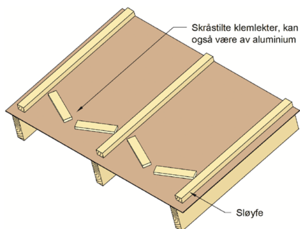
Fig. 5 Nedre klemleker skal posisjoneres skrå for å unngå vannoppsamlinger. Klemleker av stål eller aluminium er også en adekvat løsning og beskrevet i Byggforskserien.
