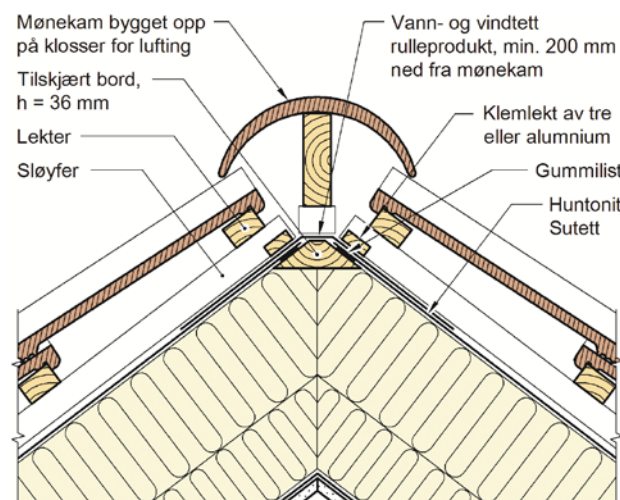
Fig. 7 Eksempel på mønedetalj. Overgangen mellom platene i de to takflatene skal gjøres lufttett ved å legge et rullbasert vindspærreprodukt som er klemt fast med klemlekte.
